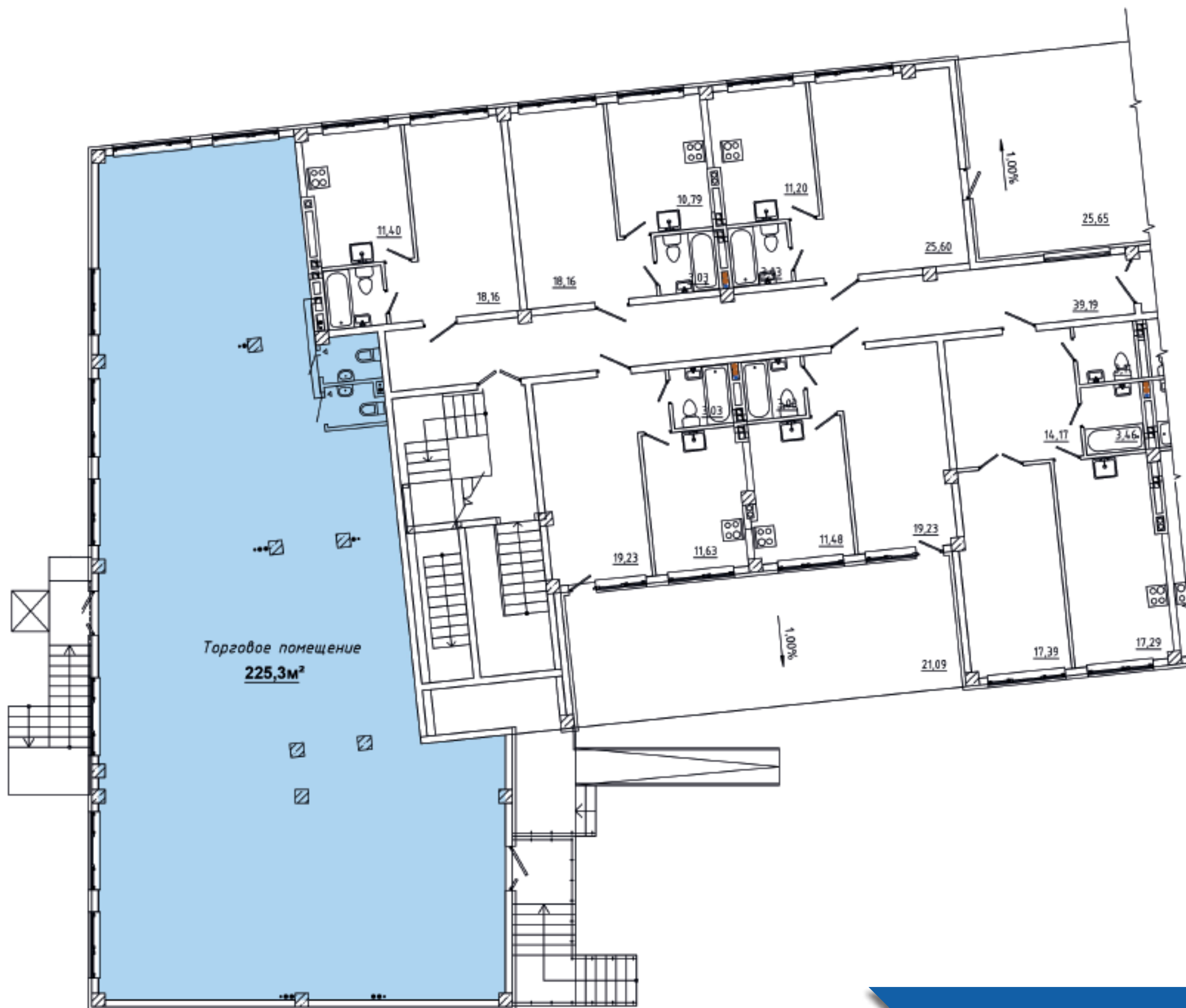
СХЕМА РАСПОЛОЖЕНИЯ БЛОКОВ
