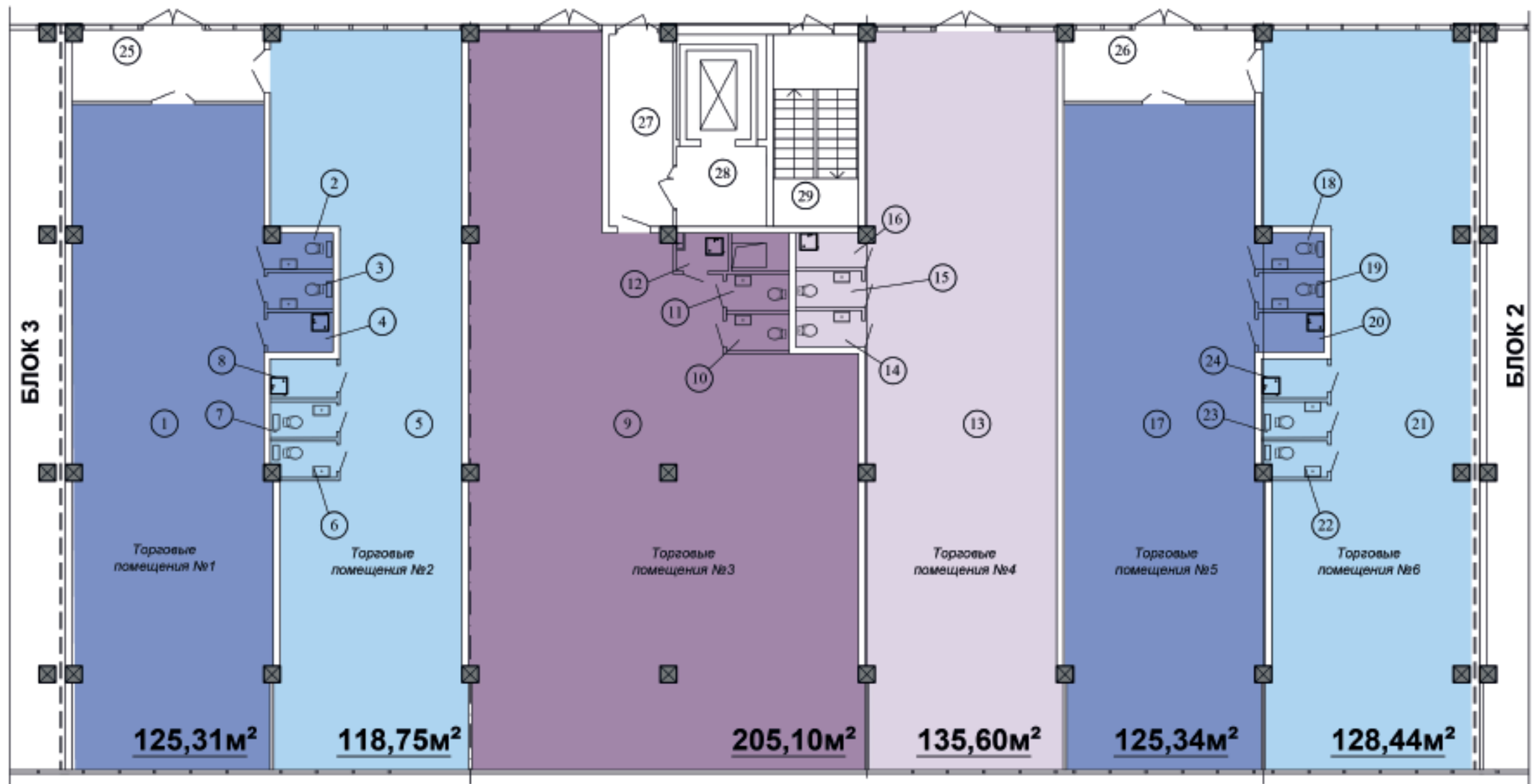
ЭКСПЛИКАЦИЯ ПОМЕЩЕНИЙ
